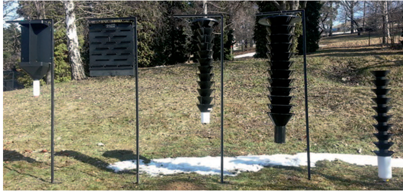
Obrázok 3. Rôzne porovnávané typy lapačov (zľava Ecotrap, Theysohn, Lindgren, lieviový prototyp, lapač BEKA)
